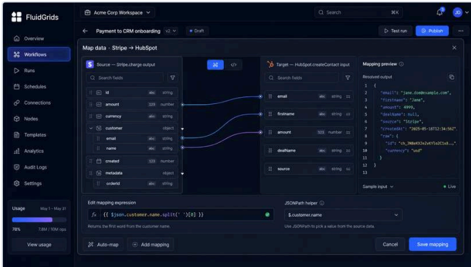
005 Fg 05 Data Mapper
