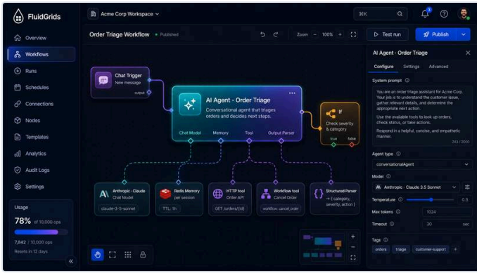
025 Fg 26 AI Agent Subnodes
